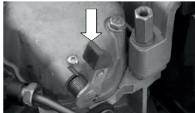
Figura 7 – Accionando la válvula de descompresión
